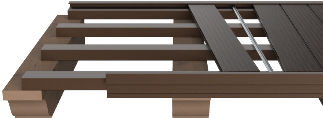
TAVOLATO A GIUNTO CHIUSO SU MAGATELLI NUOVI O PRE ESISTENTI
